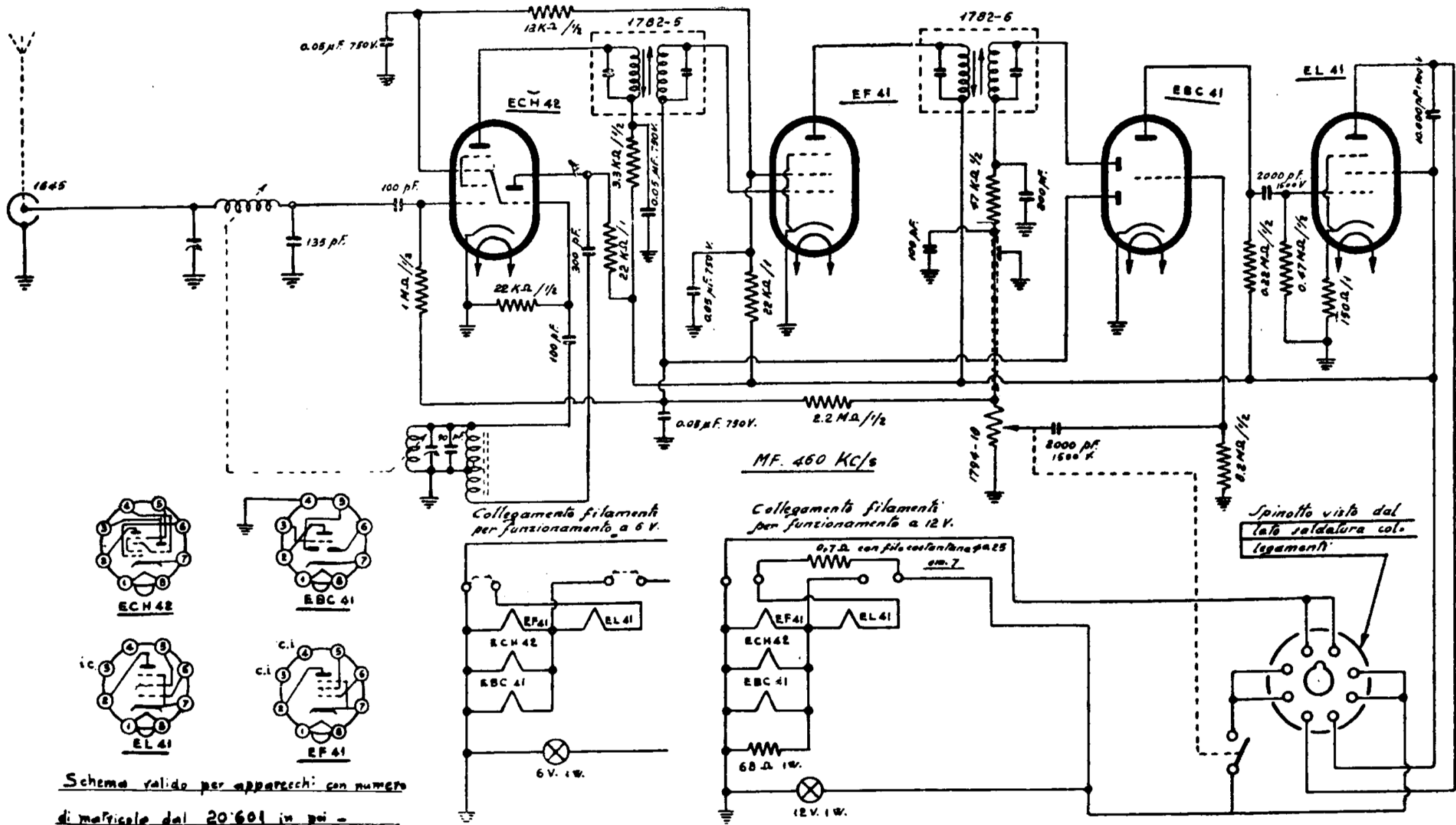
GALLO-CONDOR - Apparecchio autoradio mod. Lampo 2ª serie. Lo schema vale per gli apparecchi Lampo dal n. 20601 in poi. Media frequenza 460 kc.
